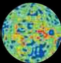
Тяготение
