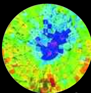
Водяной лед
