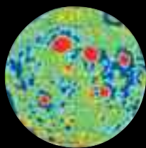
Тяготение
