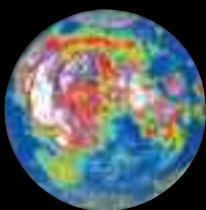
Железо
