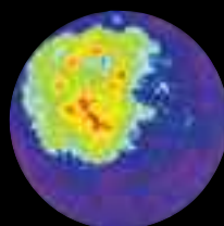
Торий
