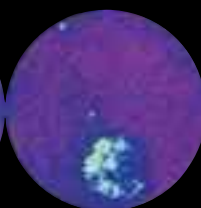
Торий
