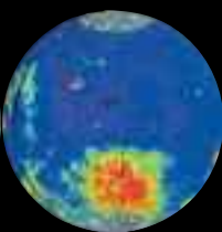
Железо
